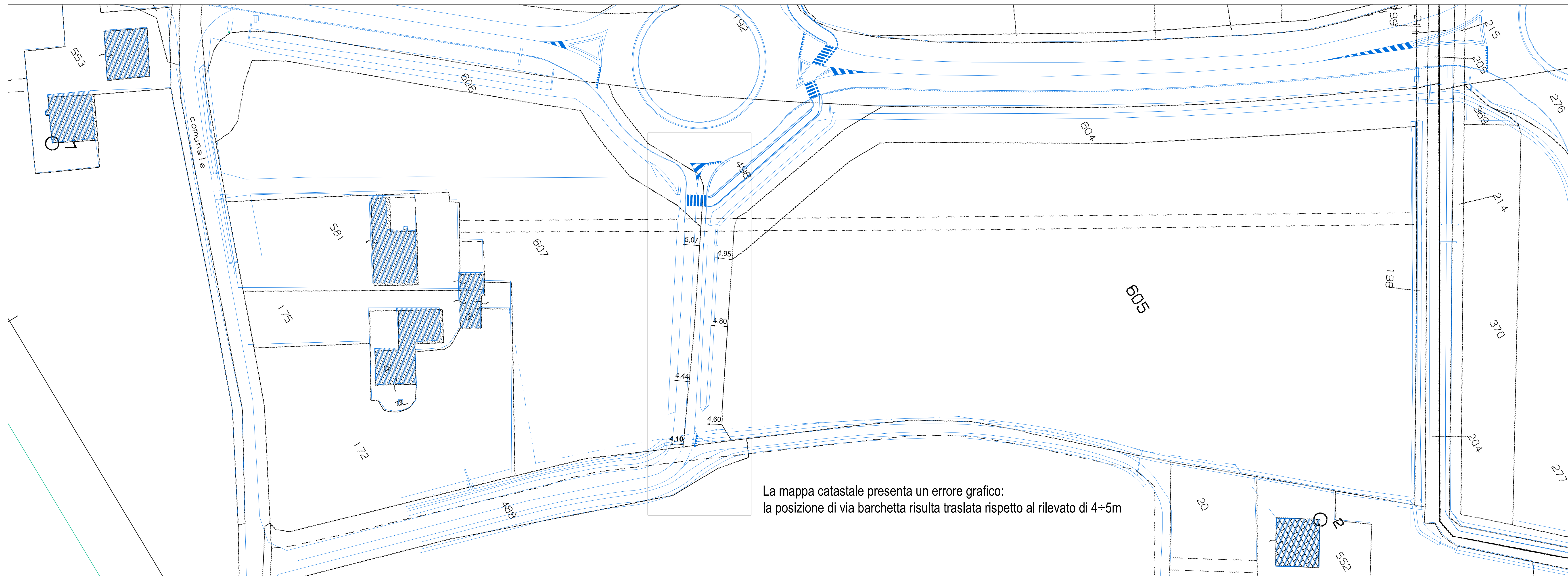
SOVRAPPONIZIONE STATO RILEVATO E MAPPA CATASTALE scala 1:1000
