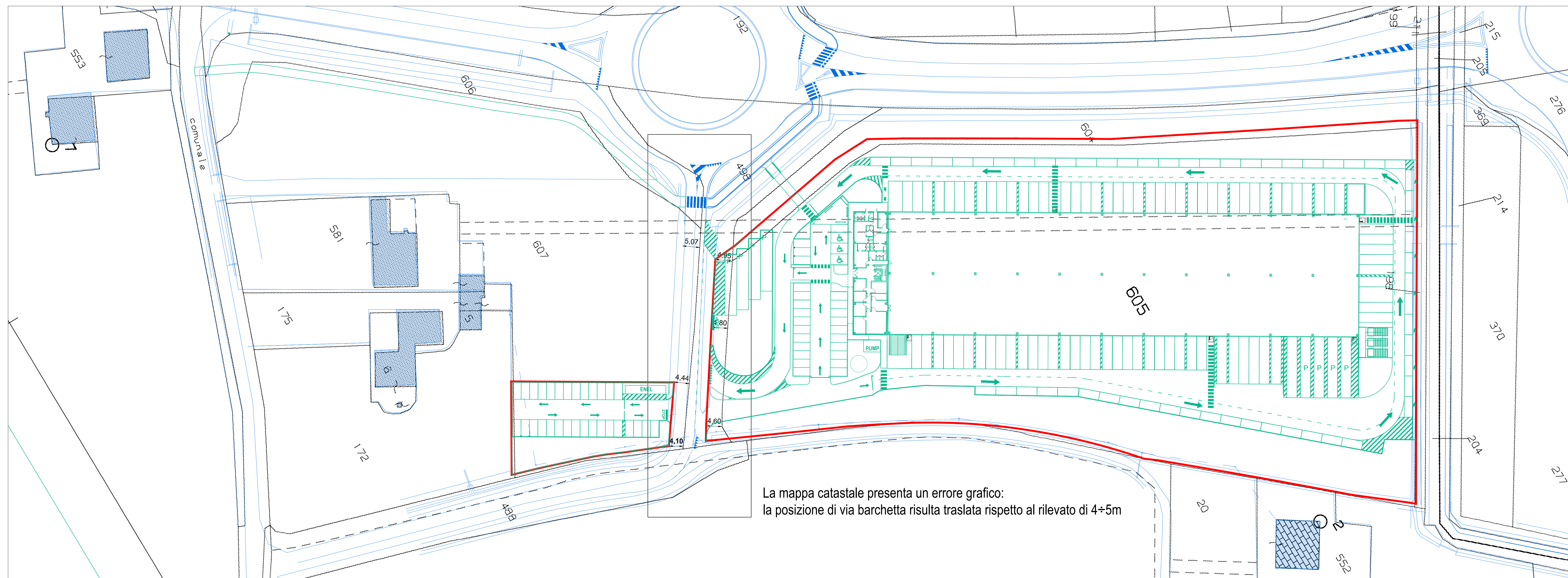
SOVRAPPONIZIONE STATO DI PROGETTO E MAPPA CATASTALE scala 1:1000
