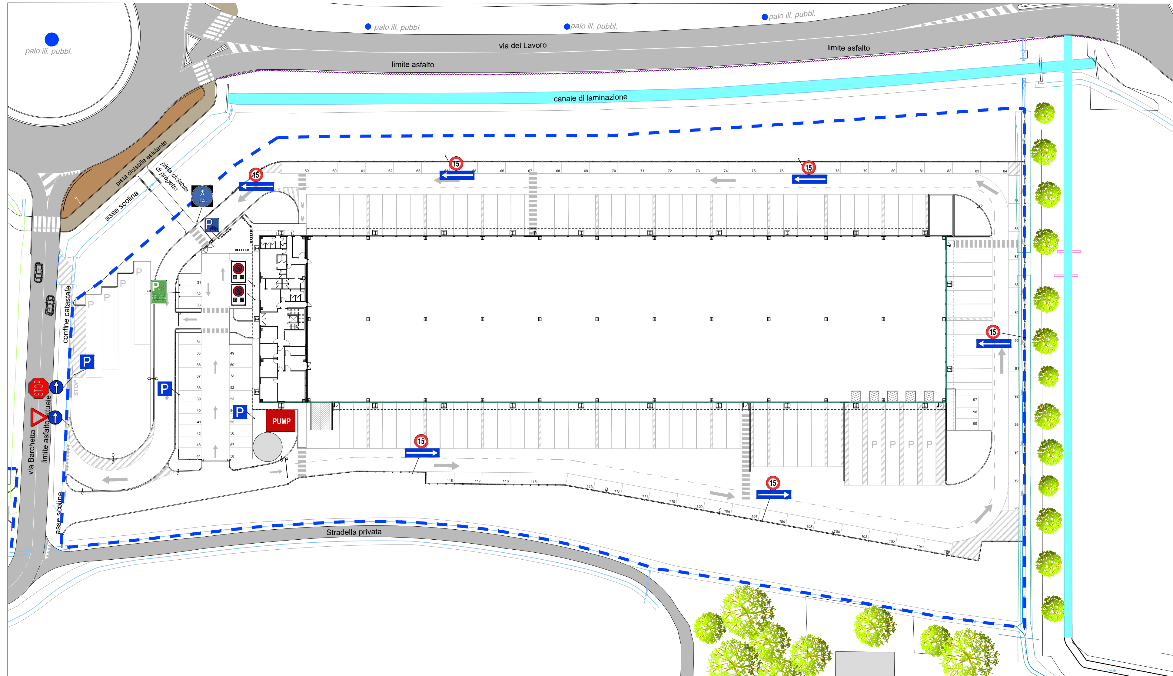
VIABILITA' E SEGNALETICA DI PROGETTO SCALA 1:500
